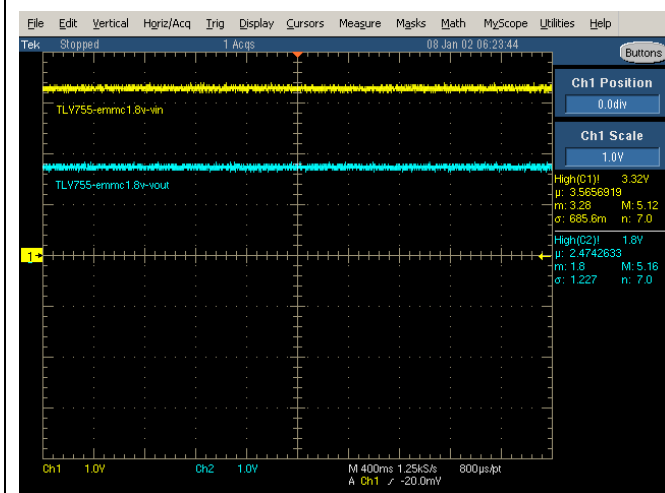
Fig. 3: Main_eMMC_VDDQ_Vin Vout
